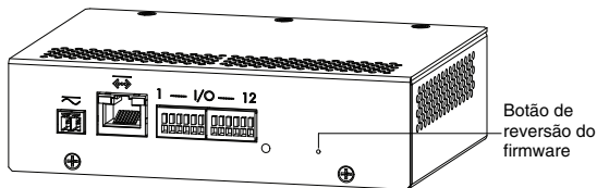
Figura: Localização do microinterruptor de reversão de firmware na parte traseira do codificador
