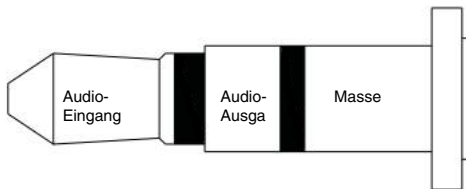
Abbildung TRS Mini-Klinkenstecker für Audio
