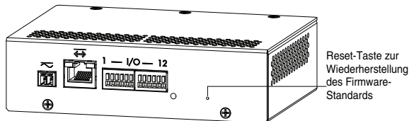
Abbildung Position des Mikroschalters zur Wiederherstellung des Firmware-Status auf der Rückseite des Encoders
