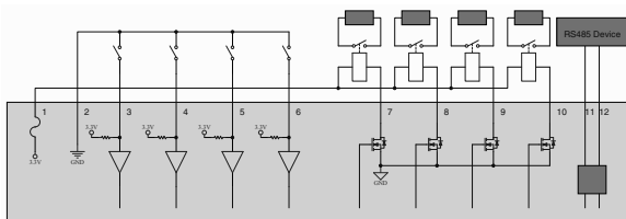
Abbildung Schaltbild des externen E/A-Terminals und Beispielanwendungen.
