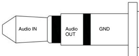
Figura : Connettore audio mini-jack TRS.
