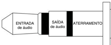
Figura: Conector de áudio minitomada TRS.
